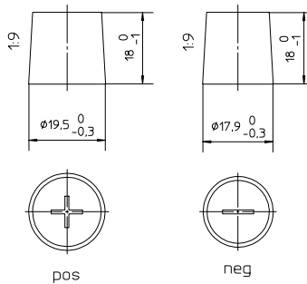
Anschlusspole 1
