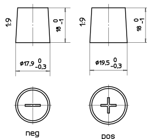
Anschlusspole 1
